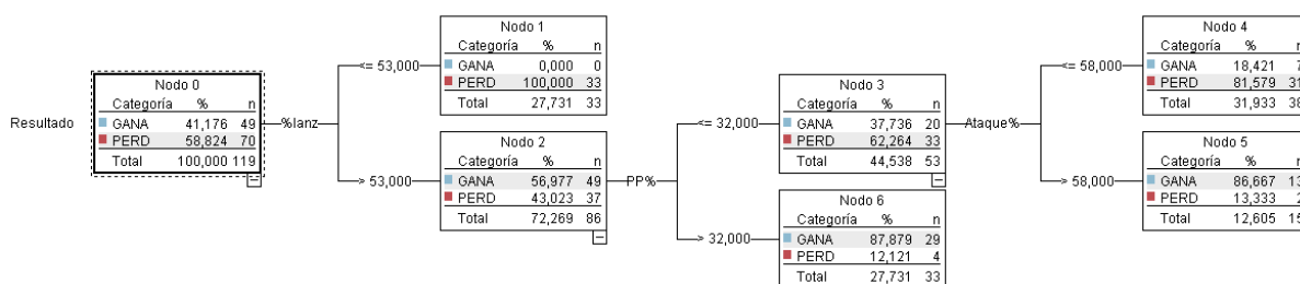
Figura 2. Configuración del árbol de decisión DT4
